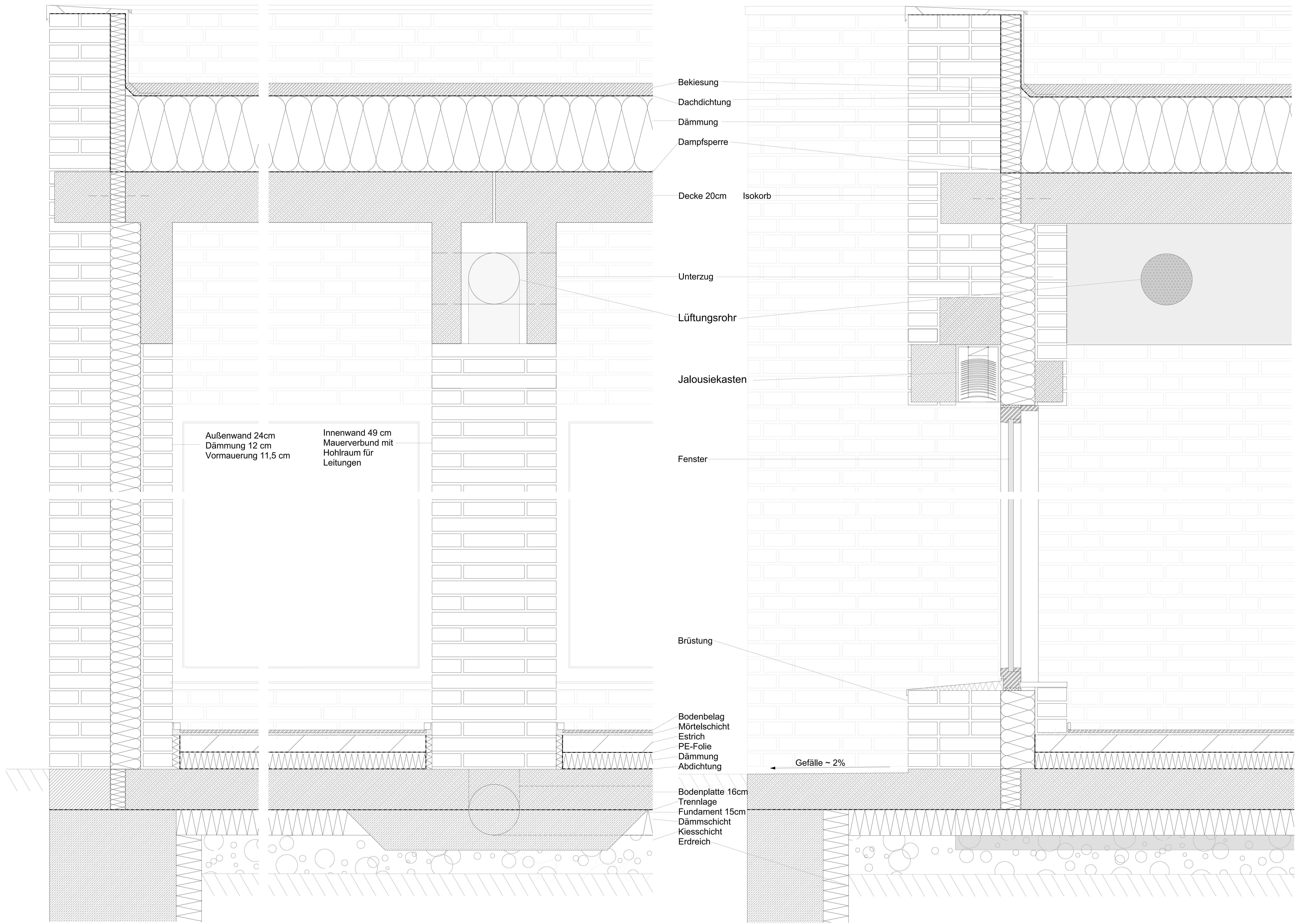
Detail 1 Außenwand Attika Wand und Bodenaufbau
